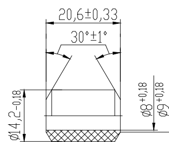
Кольцо уплотнительное (поз. 2)
